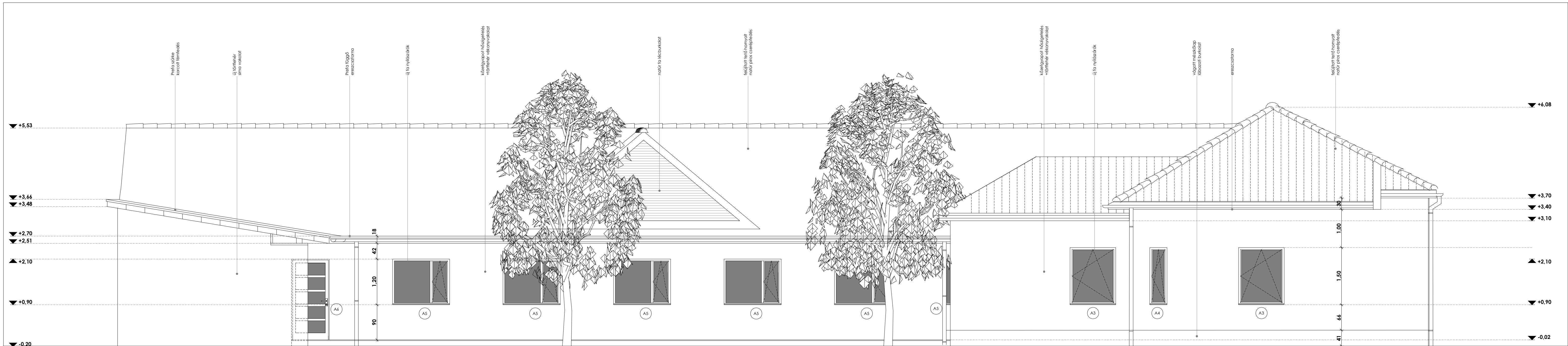
keleti homlokzat m 1:100
